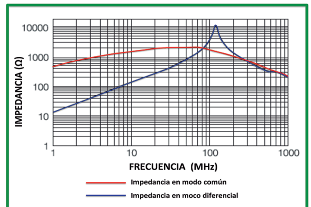
Figura 13. Impedancias de un choque en modo común con devanado separado.
