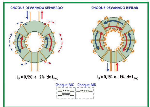
Figura 12. Inductancia de fuga ( L_f ) (inductancia en MD) como porcentaje de la inductancia en modo común ( L_{MC} ).
