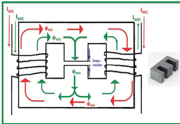
Figura 10. Caminos del flujo magnético en modo común (MC) y en modo diferencial (MD) en un choque con núcleo tipo "E". La separación central controla la inductancia L_{DM} .
