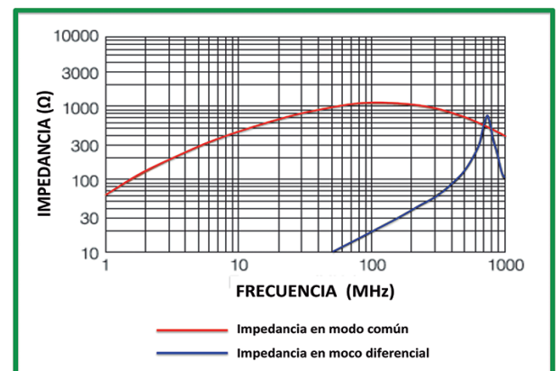
Figura 14. Impedancias de un choque en modo común con devanado bifilar.
